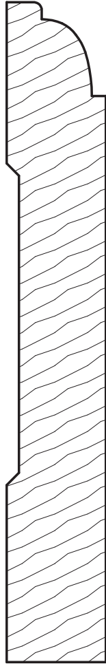
SEB-222 3/4 x 5
