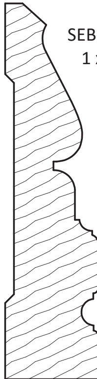
SEB-162 13/16 x 4-1/4
