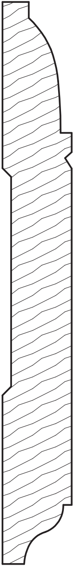
SEC-242 3/4 x 6
