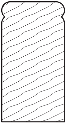
LOU-008 1-1/16 x 2
