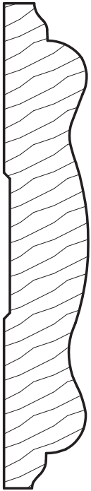
SEH-071 5/8 x 3-9/16
